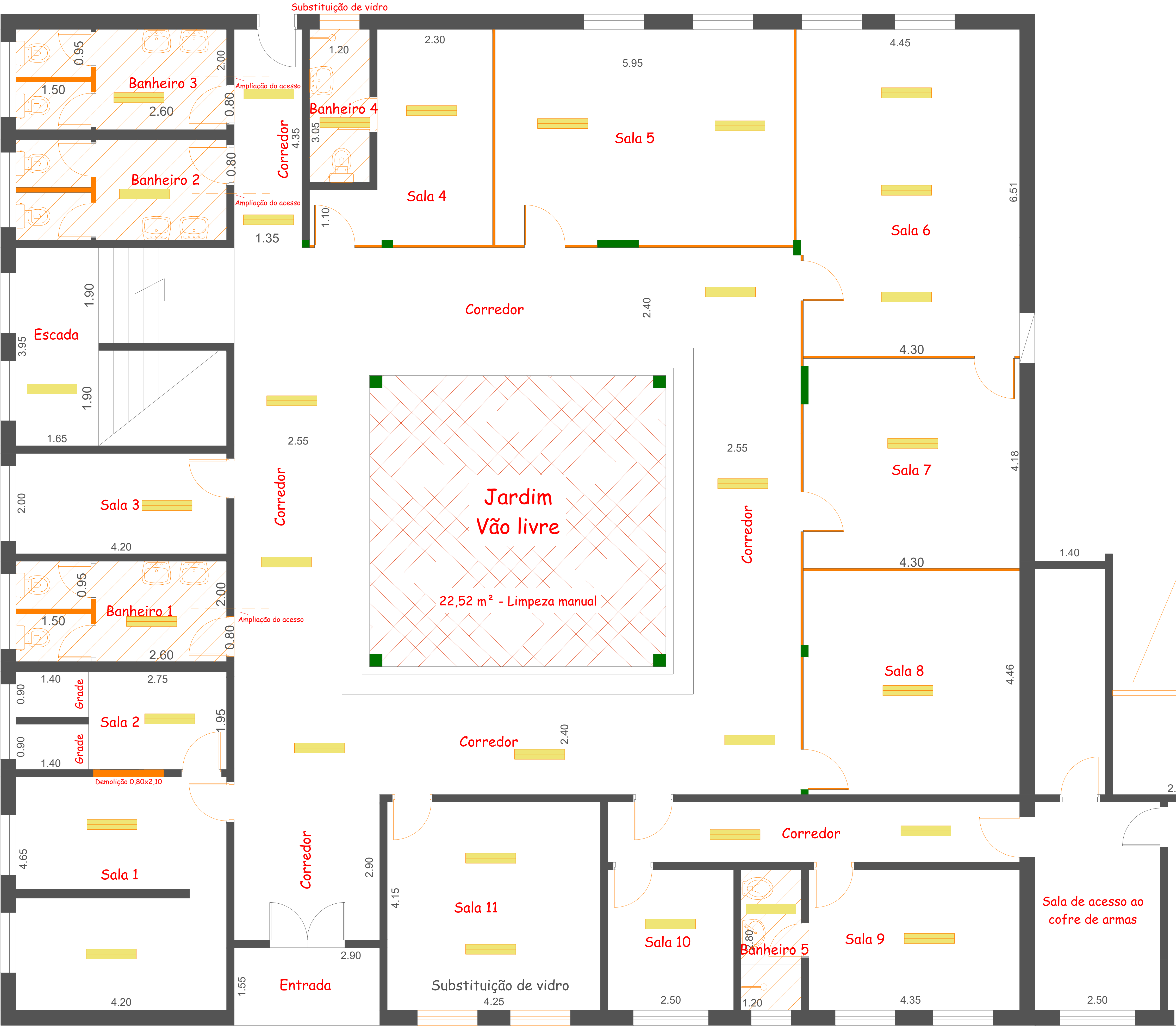
PLANTA DE DEMOLIÇÃO INTERNA TÉRREO SEM ESCALA
