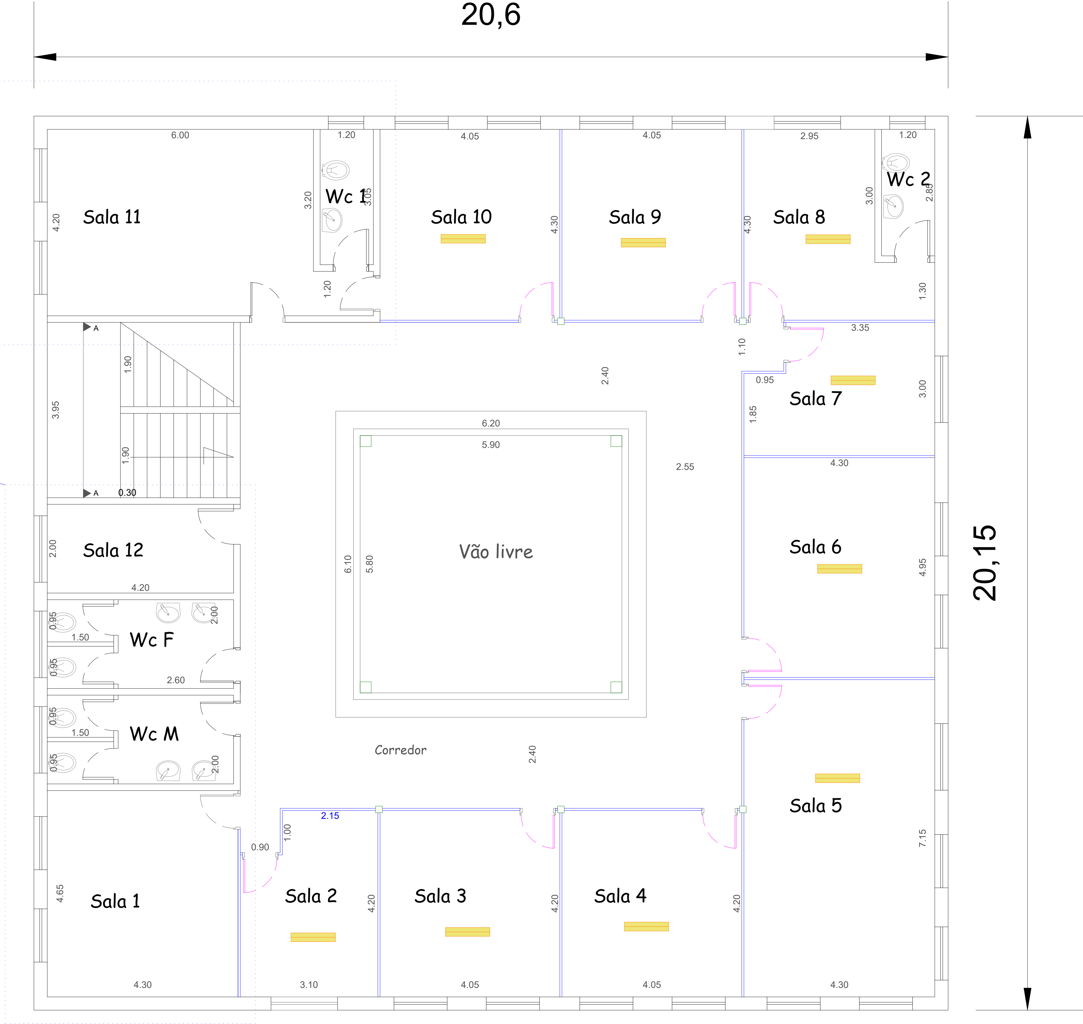
PLANTA DO SEGUNDO ANDAR SEM ESCALA
