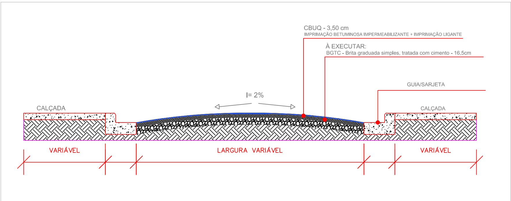
DETALHAMENTO A – CORTE AA S/ ESCALA
