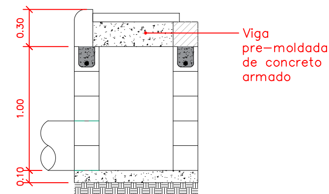
DETALHAMENTO C - CORTE BB
