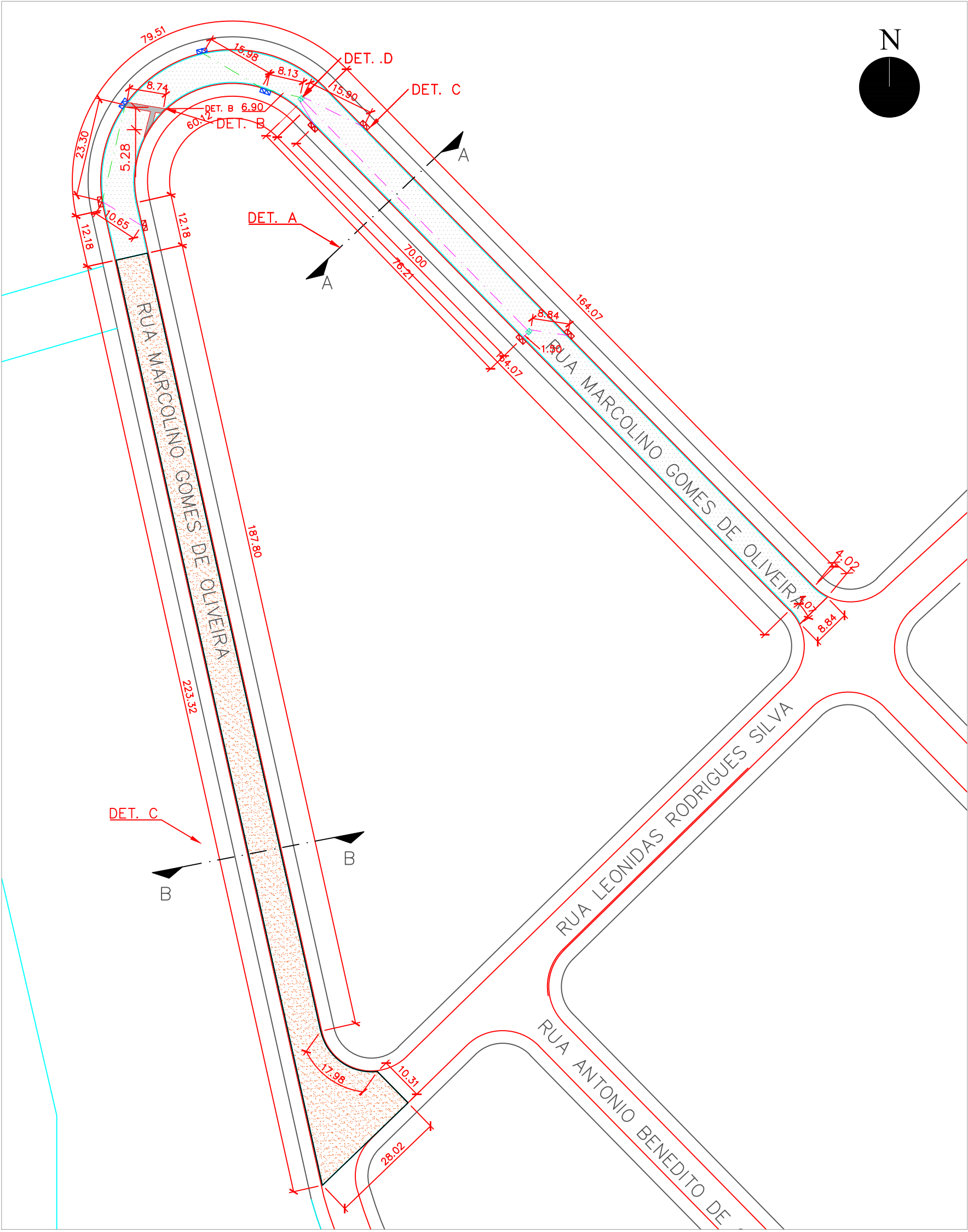
PLANTA – TRECHO 1 ESCALA 1/975
