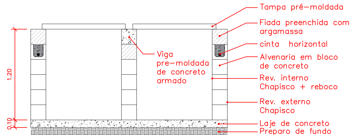
DETALHAMENTO C - CORTE AA
