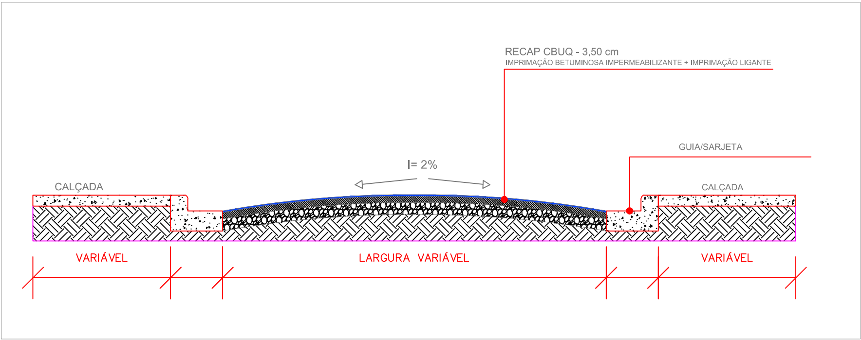
DETALHAMENTO C – CORTE BB S/ ESCALA
