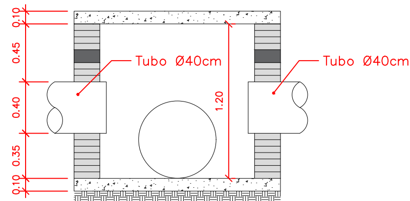
DETALHAMENTO D - CORTE BB
