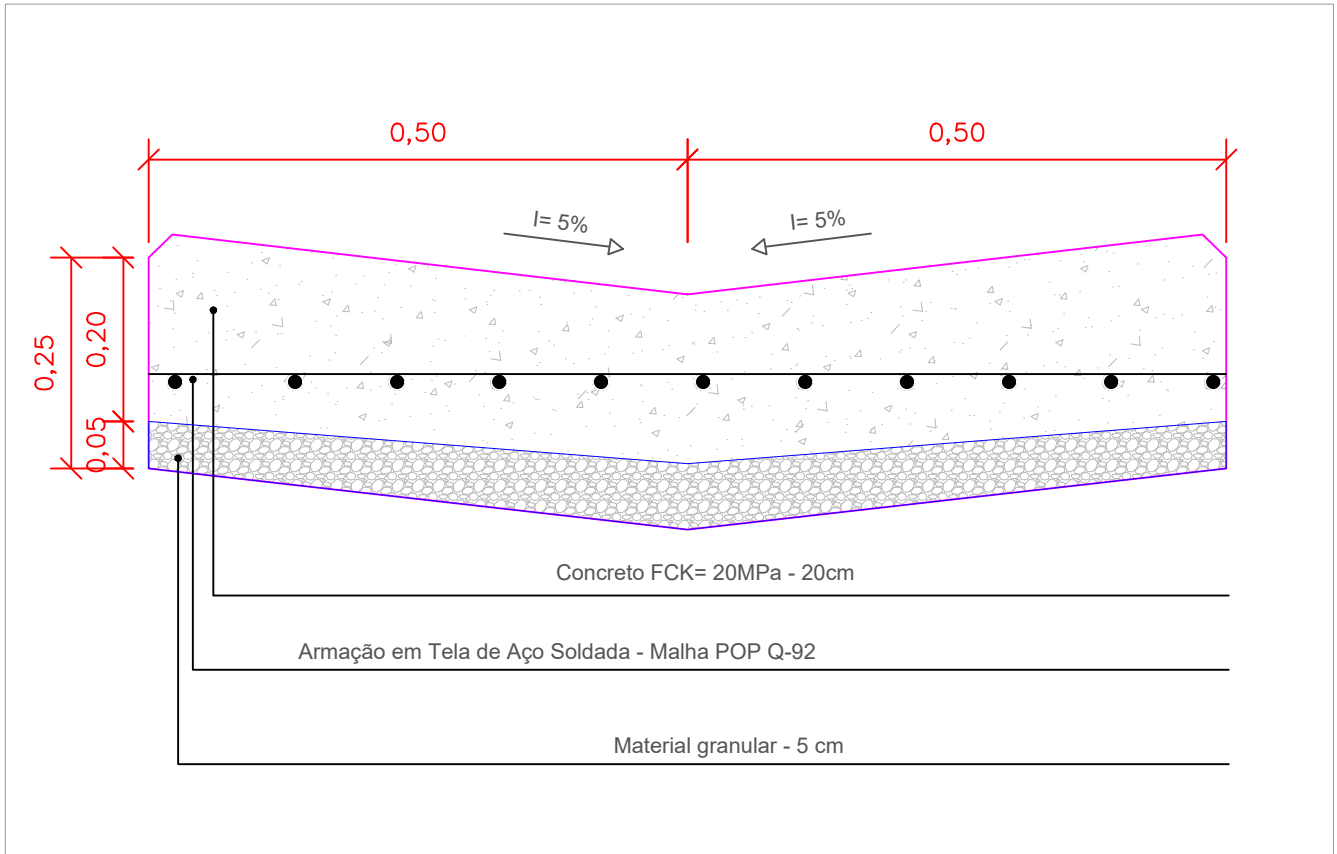
DETALHAMENTO B S/ ESCALA
