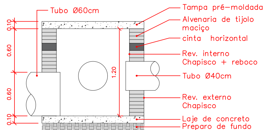
DETALHAMENTO D - CORTE AA
