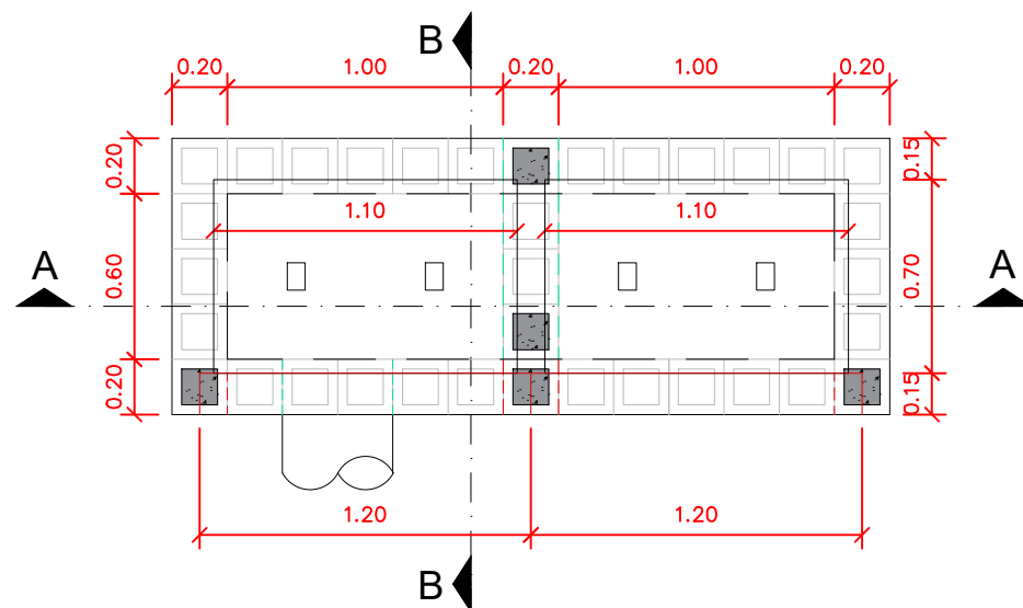
DETALHAMENTO C - PLANTA
