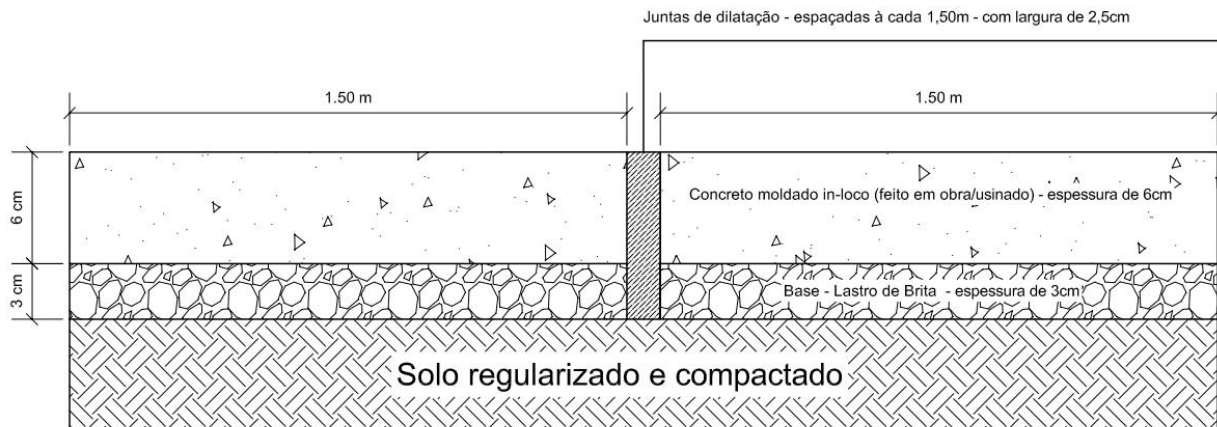
Detalhe da calçada - sem escala
