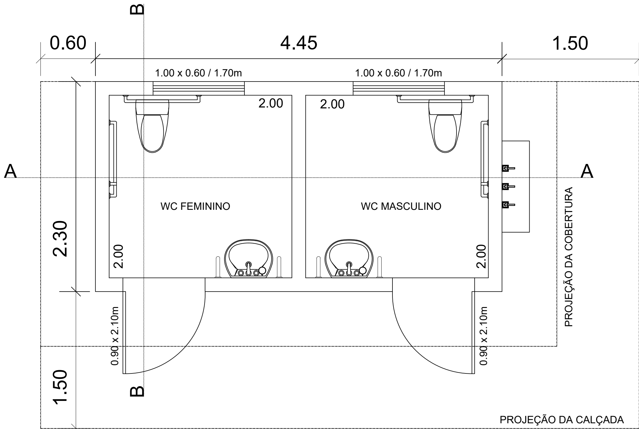
PLANTA BAIXA - Esc. 1/25
