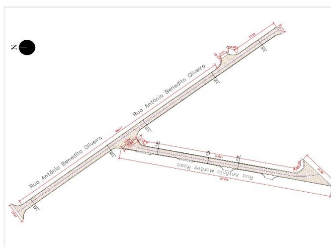
PLANTA GERAL ESCALA 1/1300
