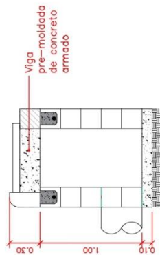
DETALHAMENTO C - CORTE BB
