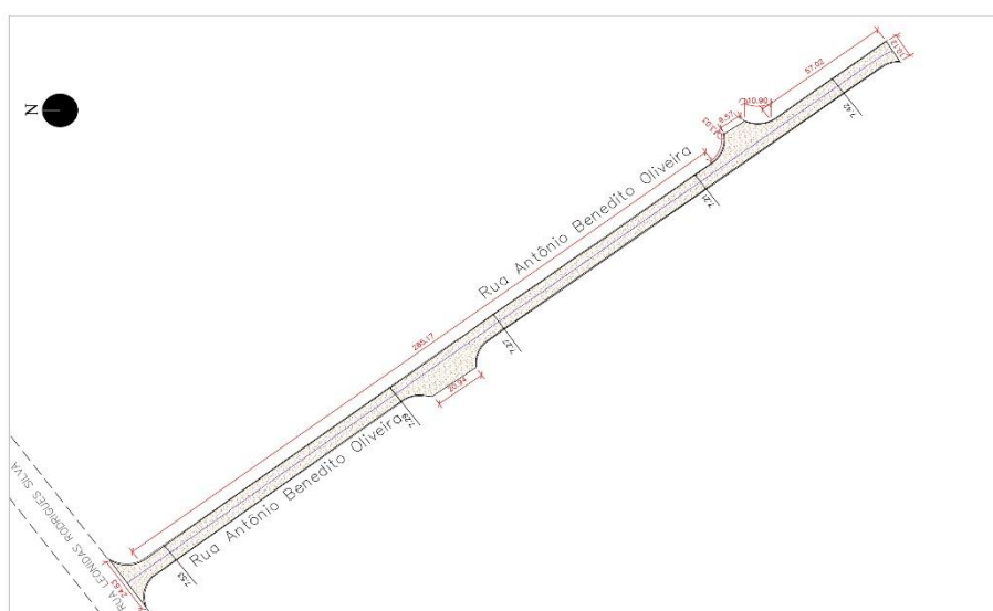
PLANTA - TRECHO ANTÔNIO BENEDITO OLIVEIRA ESCALA 1/975
