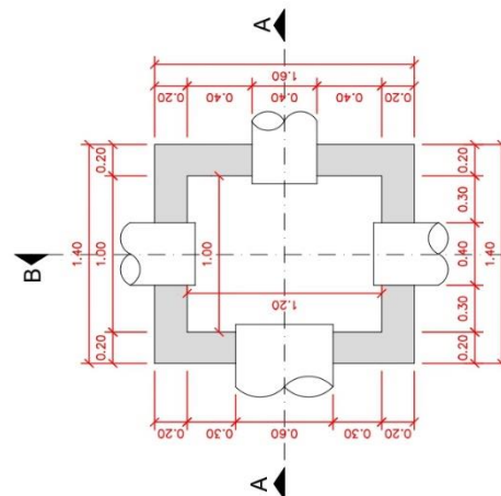
DETALHAMENTO D - PLANTA
