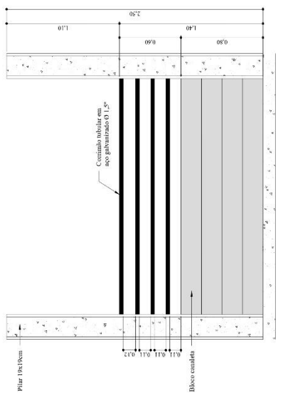
DETALE GUARDA-CORPO S/ escala
