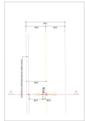
DET. 01 - PLANTA - ESCALA: 1/2800
