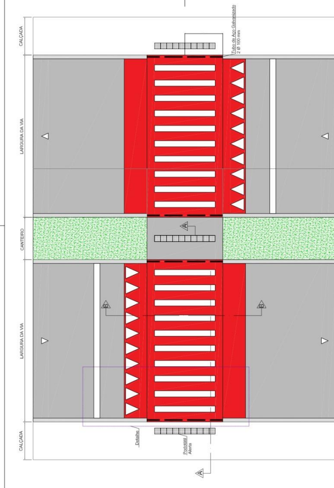
IMPLANTAÇÃO ESC. 1:100
