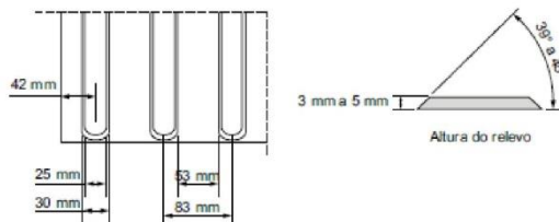
Figura 13 - Dimensionamento dos relevos do piso tátil direcional
