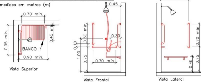
Figura 10 - Dimensões boxe para chuveiro acessível
