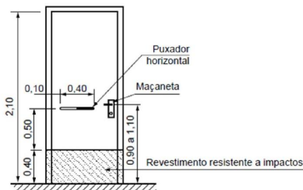
Figura 4 - Sinalização e comunicação em portas
