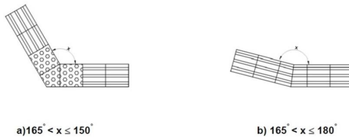
Figura 14 - Exemplos de mudança de direção
