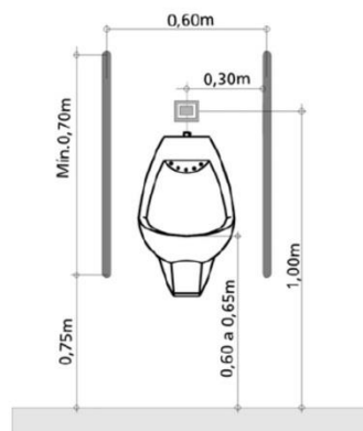
Figura 9 - Dimensões Mictório
