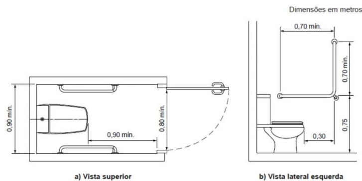
Figura 7 - Boxe com barra de apoio
