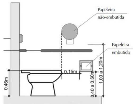
Figura 6 - Dimensões bacia sanitária e papeleira
