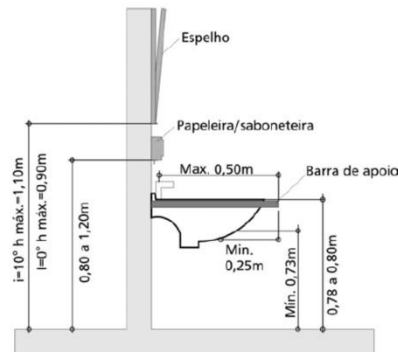
Figura 8 - Dimensões lavatório
