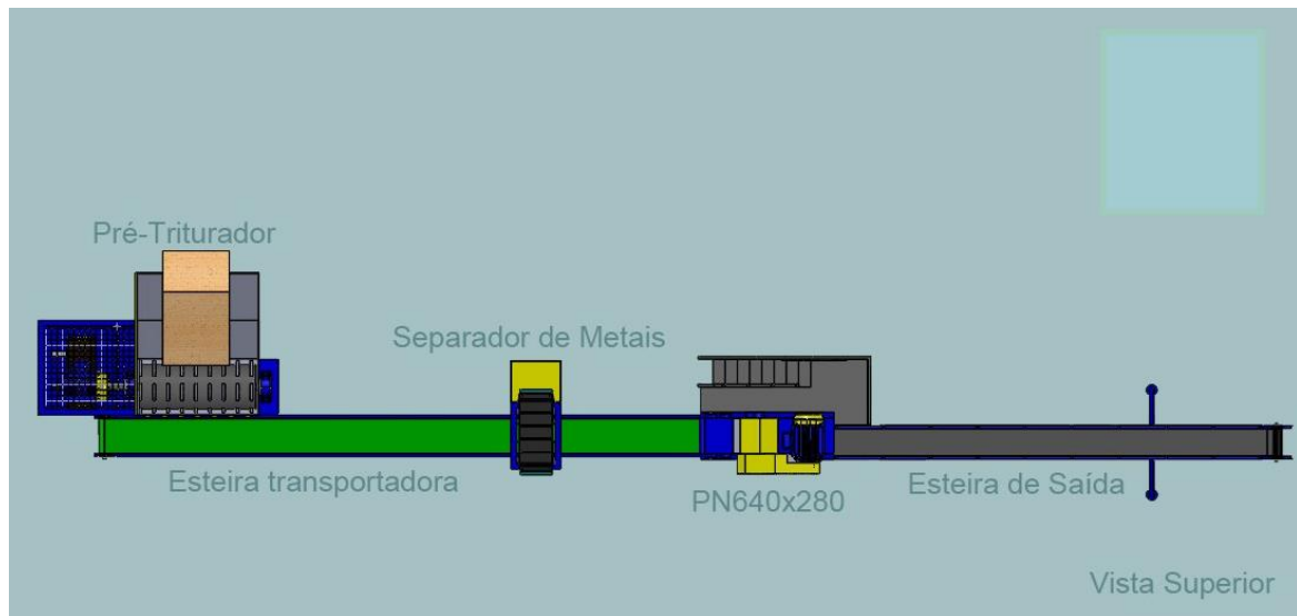
Fig.3: Vista superior do processo.
